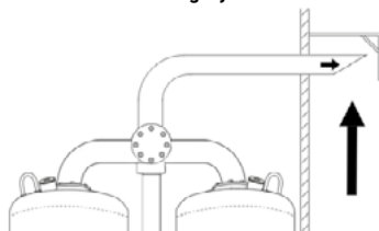
Osłona atmosferyczna przy bocznym ułożeniu przewodu
