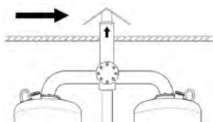
Osłona atmosferyczna przy ułożeniu przewodu do góry
