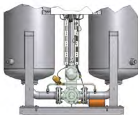
Wlot sprężonego powietrza do osuszacza
