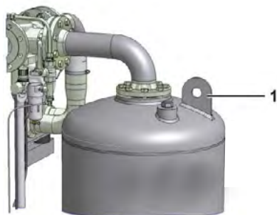
Zaczepy do podnoszenia / Zaczepy do mocowania
