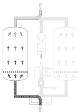
Adsorpcja przebiegająca w lewym zbiorniku
